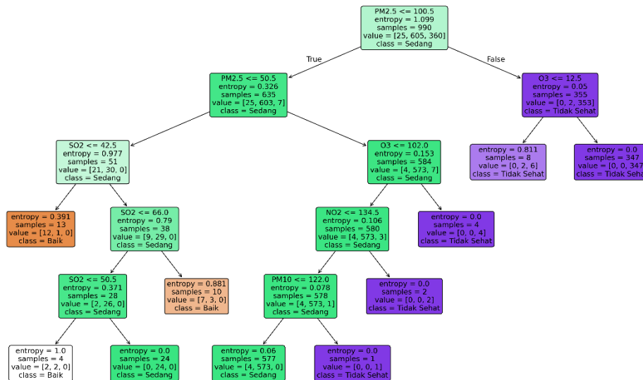
Gambar 2. Pohon Keputusan
